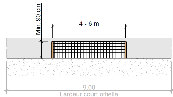
COUPE
