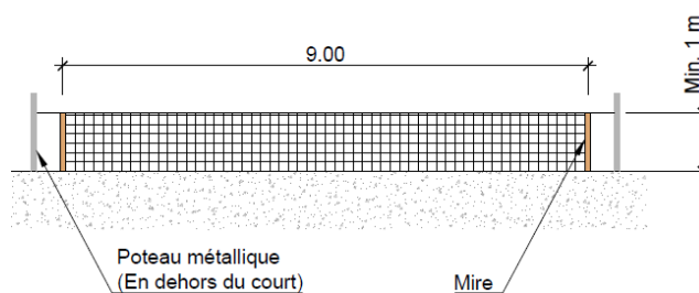
COUPE
