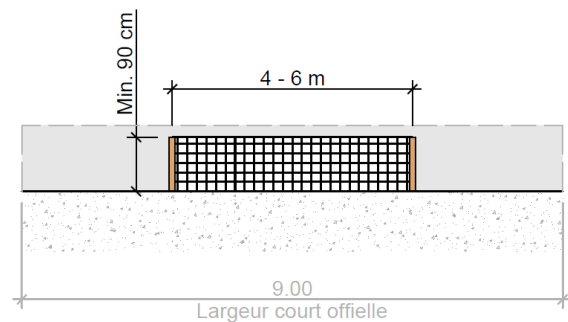
COUPE
